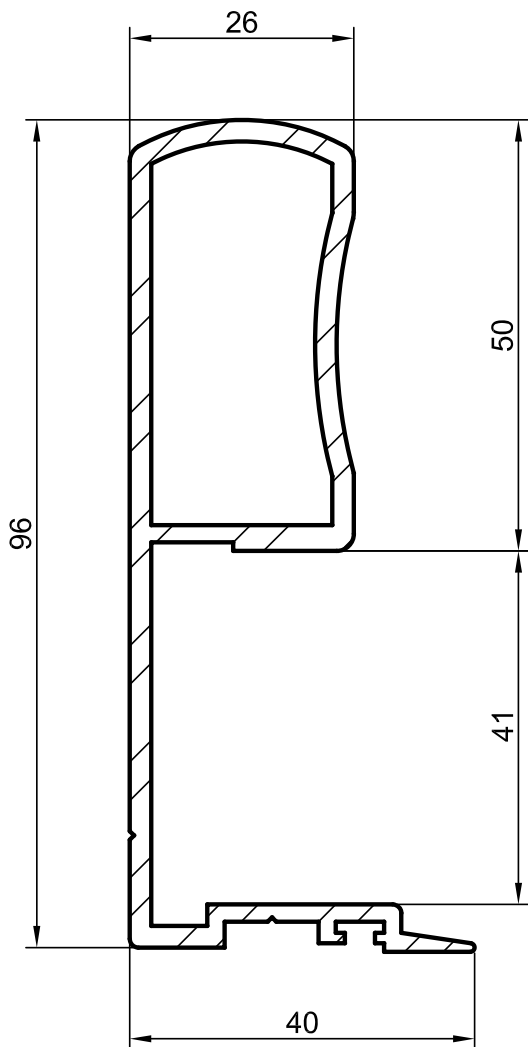
Профили среднего стыка и крышек
