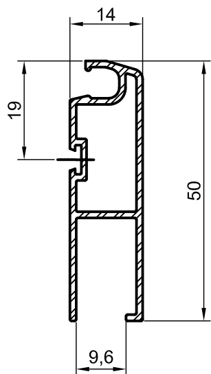
Рамка москитной сетки (алю.)
